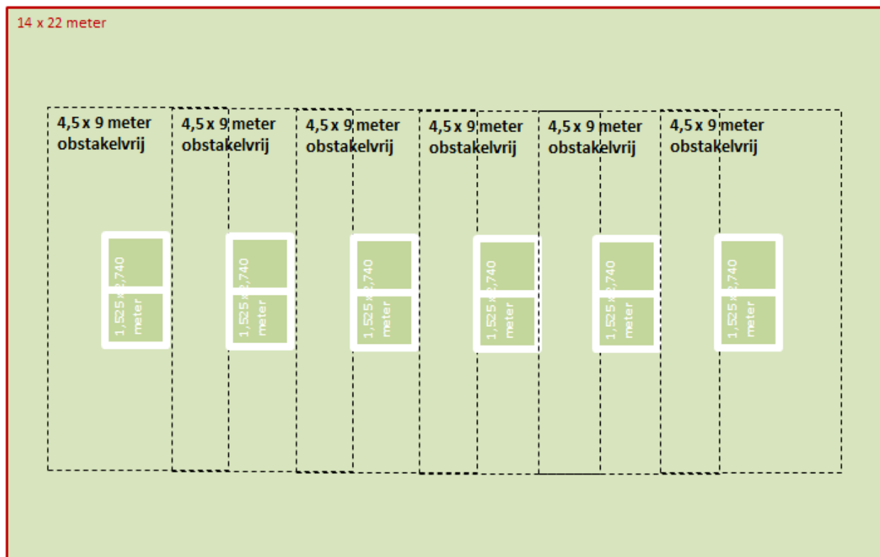
Figuur 1: Tafeltennis; 6xwedstrijdopstelling afdelingsklasse (inclusief obstakelvrije uitloop). De hoogte van 5,5 meter volstaat ruimschoots (minimaal 4 meter).
