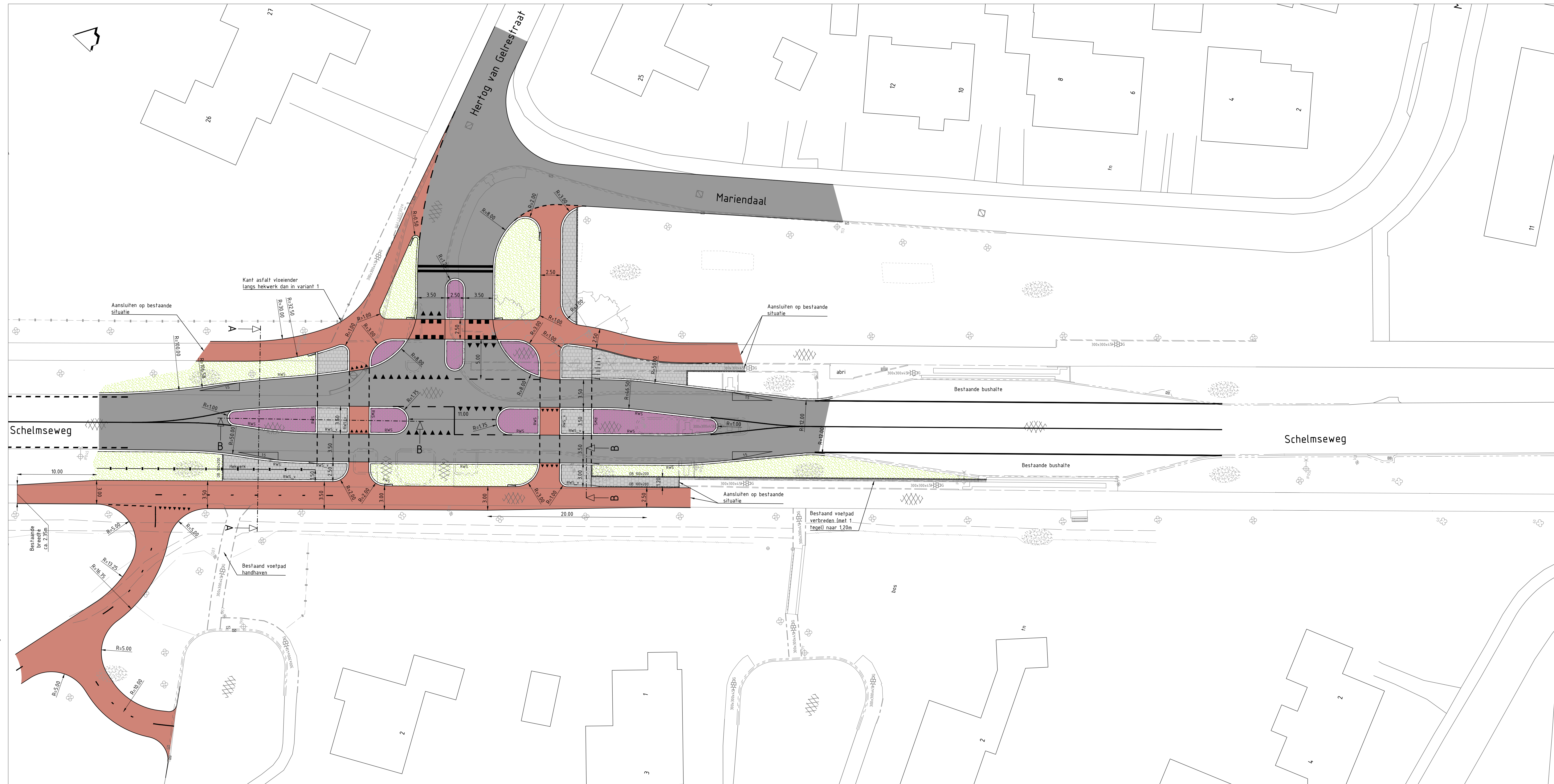
Oversteek Variant 1 met 3,50m middenberm i.p.v. 4,00m (SCHAAL 1:200)
